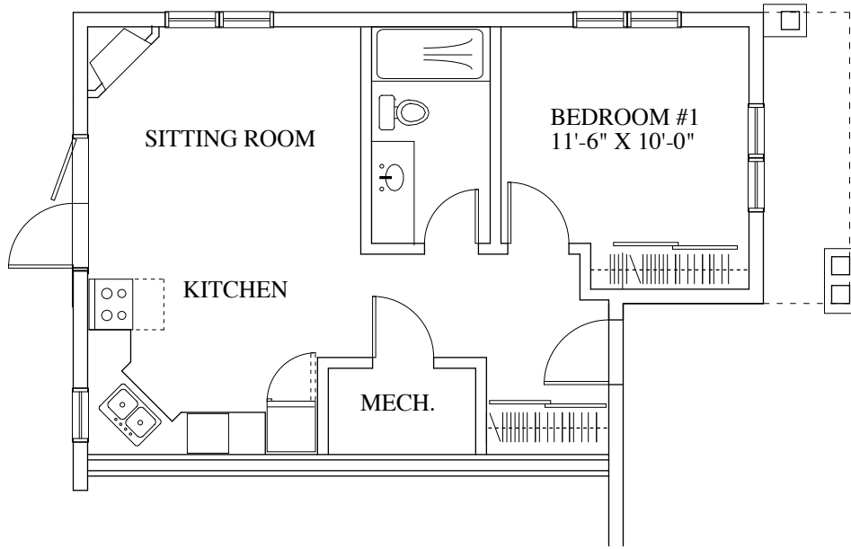
1 UNIT 9 - MAIN A9 SCALE: 1/4" = 1'-0"
