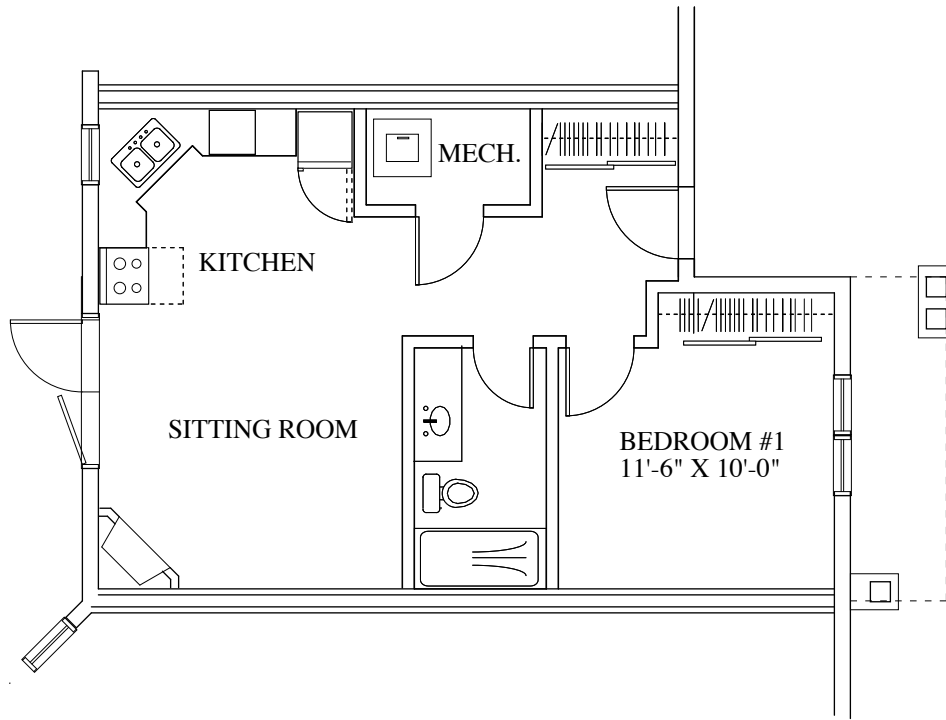
1 UNIT 8 - MAIN A8 SCALE: 1/4" = 1'-0"
