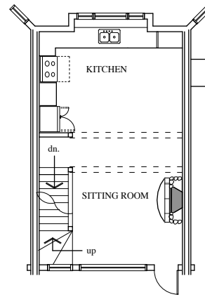
2 UNIT 5 - SECOND A5 SCALE: 1/8" = 1'-0"
