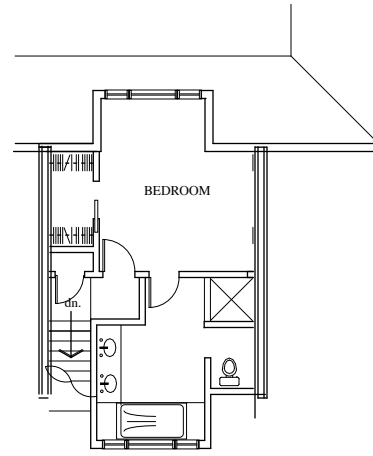
2 UNIT 5 - SECOND A5 SCALE: 1/8" = 1'-0"
