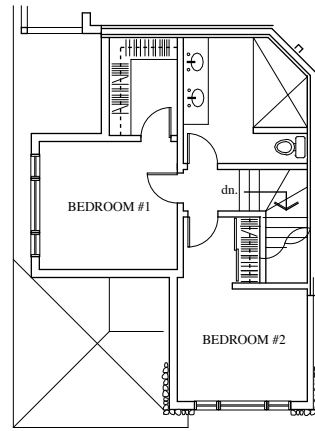
2 A3 UNIT 3 - SECOND SCALE: 1/8" = 1'-0"
