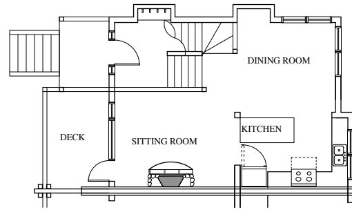
2 UNIT 1 - SECOND A1 SCALE: 1/8" = 1'-0"
