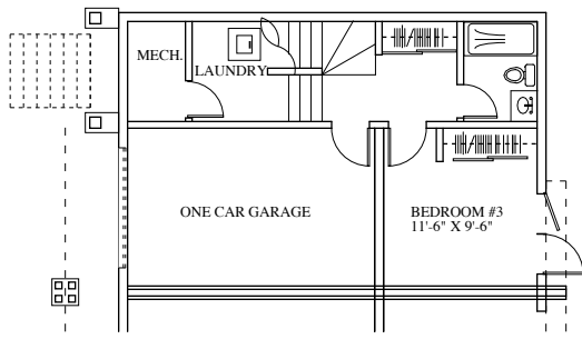
1 UNIT 1 - MAIN A1 SCALE: 1/8" = 1'-0"
